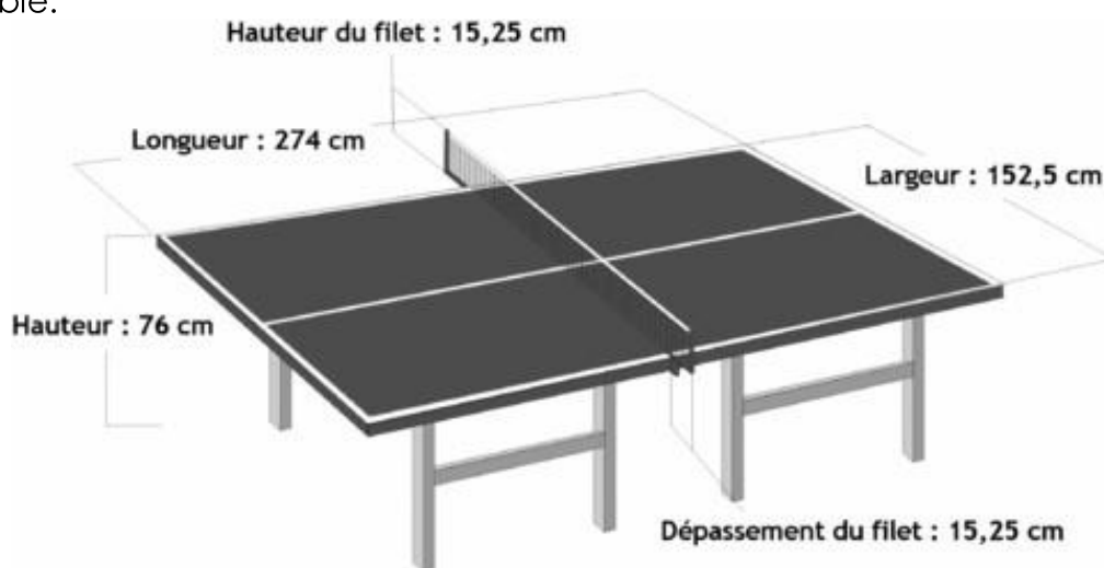
Dimensions de la table de tennis de table.
